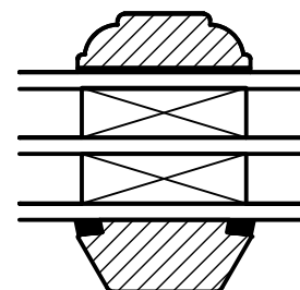
Fig. 8 42 mm. BONDEHUSPROFIL 42 mm. FARMHOUSEPROFILE 42 mm. PALASTSPROSSEN
