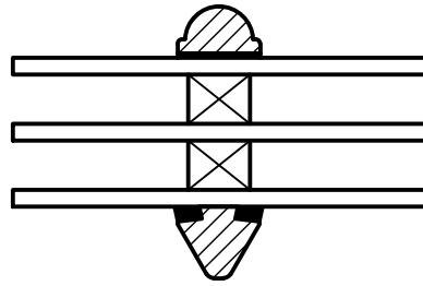
Fig. 2 20 mm. BONDEHUSPROFIL 20 mm. FARMHOUSEPROFILE 20 mm. PALASTSPROSSEN
