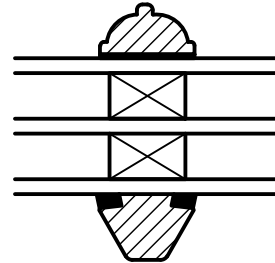
Fig. 4 25 mm. BONDEHUSPROFIL 25 mm. FARMHOUSEPROFILE 25 mm. PALASTSPROSSEN
